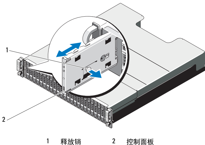
图 16-14. 卸下和安装控制面板 -PowerVault MD3620f
